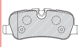
FDB1613 TRW 24192 116.6 x 46.5 x 17.3mm
