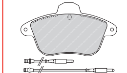
FDB1070 CIT 23161 83 x 75 x 15.3mm
