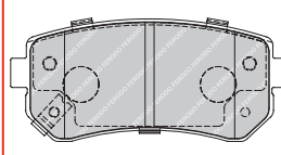
FDB1956 MAN 24320 93.2 x 41.1 x 16mm
